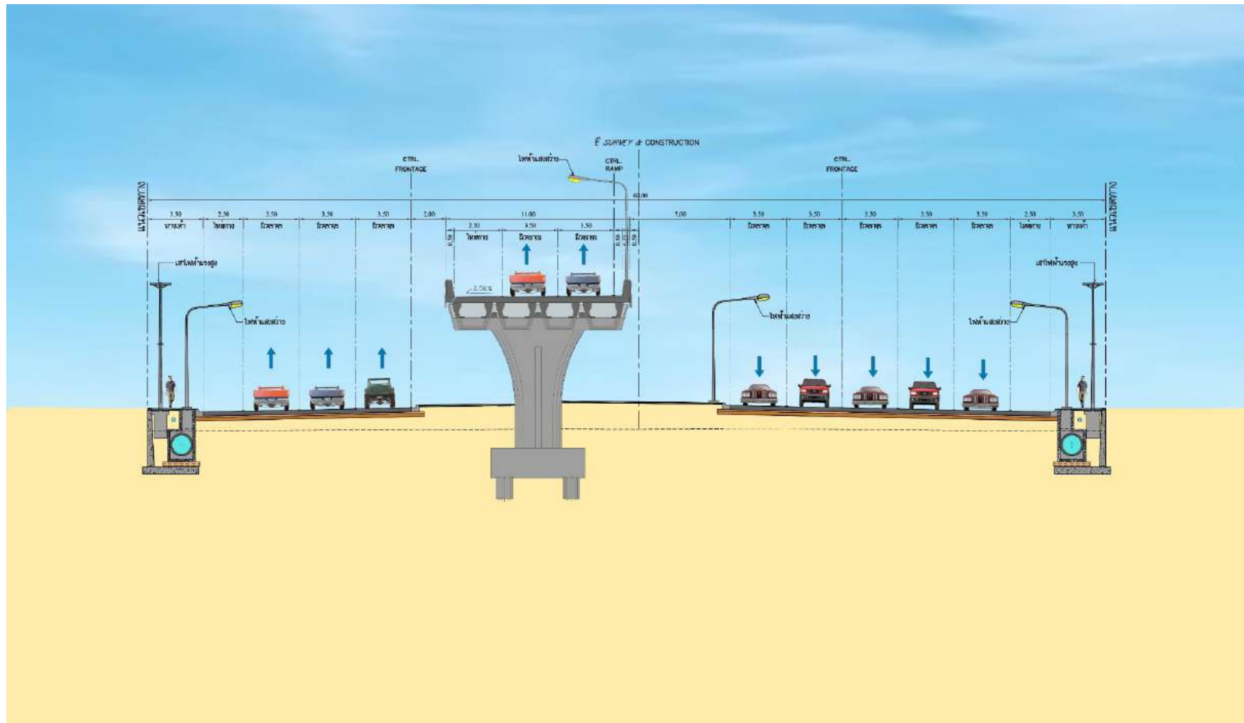
รูปที่ 6.1-3 รูปตัดทั่วไปถนนโครงการช่วงที่ 1 งานออกแบบทางแยกต่างระดับ
