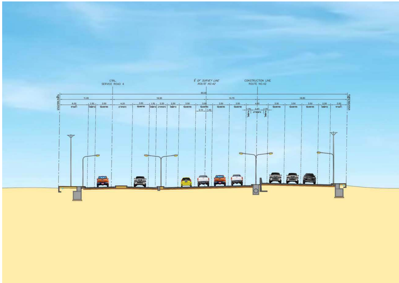
รูปที่ 6.1-5 รูปตัดทั่วไปถนนโครงการช่วงที่ 2 ออกแบบปรับปรุงถนนโครงการ
